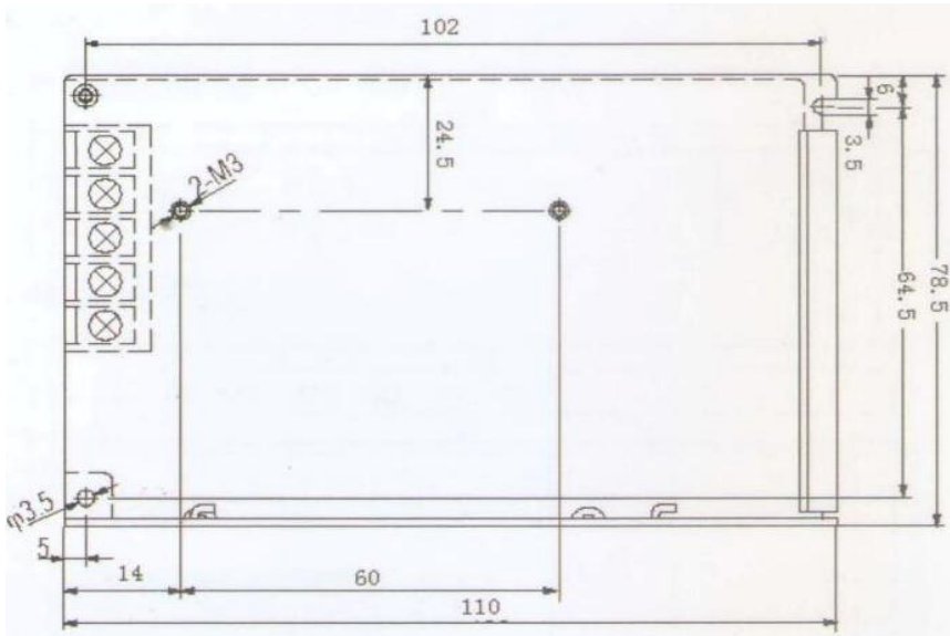
机构尺寸图：
