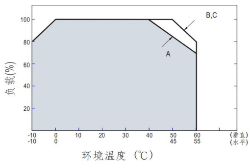
降额曲线：
