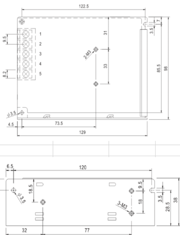
■ 机构尺寸
