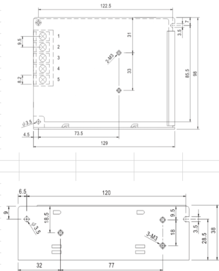
■ 机构尺寸
