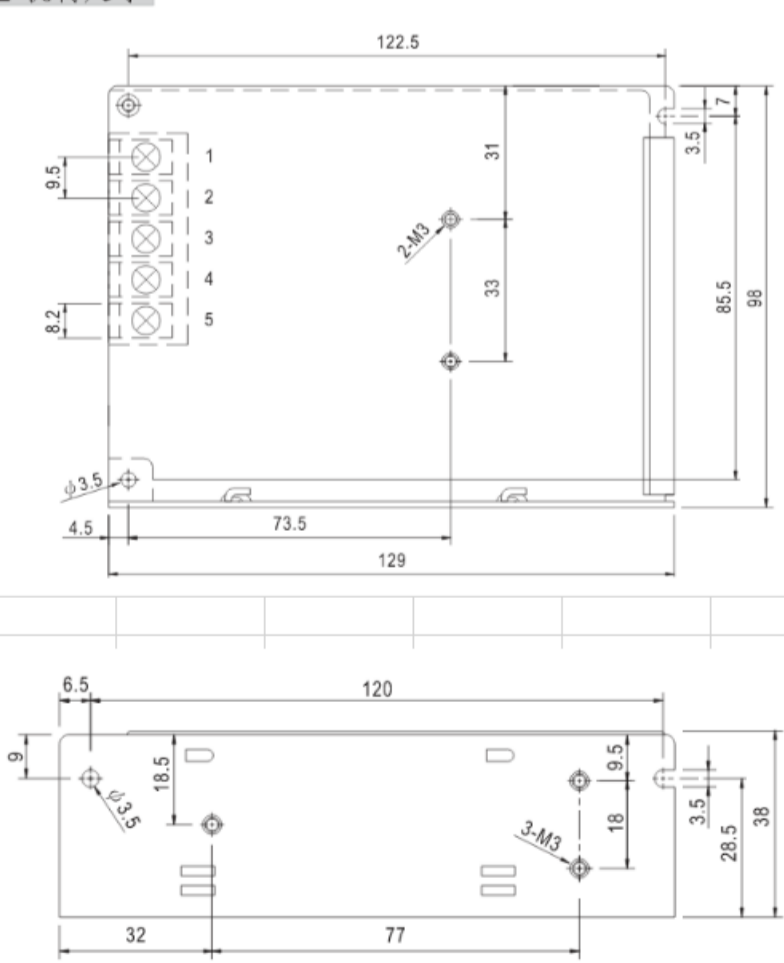
■ 机构尺寸
